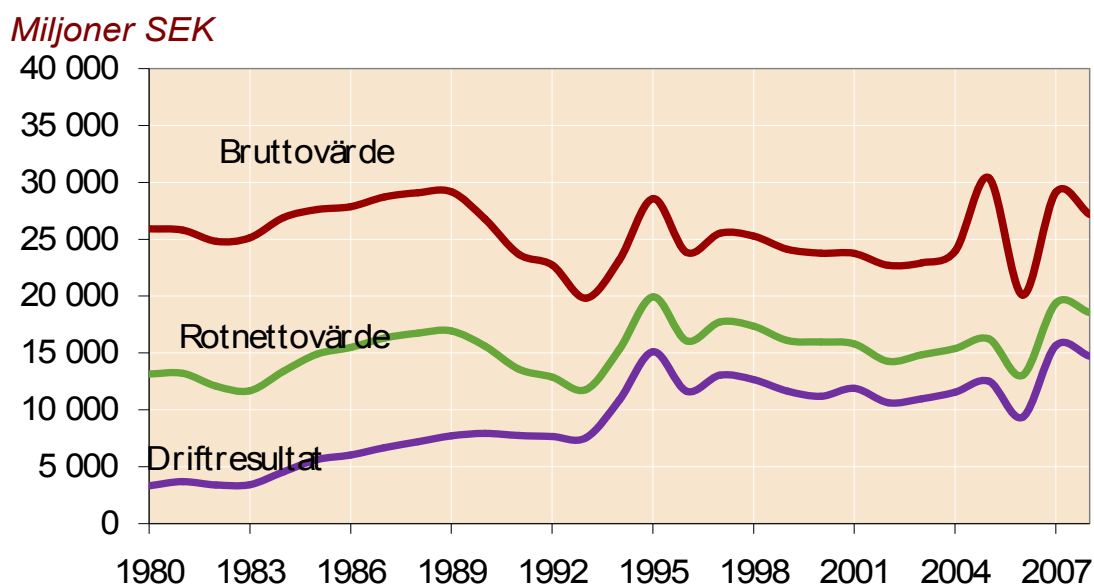
Figur 4: Avverkningarnas brutto-, rotnetto- och driftresultatsvärden, i 2008 års prisnivå (deflaterat med KPI)
